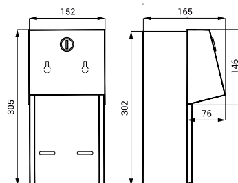
SLZN 26Z 95261 Dispenser de hârtie igienică din oțel inox încastrat
