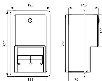
SLZN 37 95370 Dispenser de hârtie igienică din oțel inox
